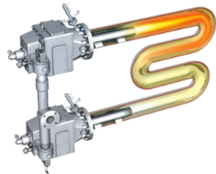
リージェネレイティブバーナー
